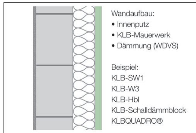
Einschaliges Mauerwerk mit Dämmung (WDVS)
