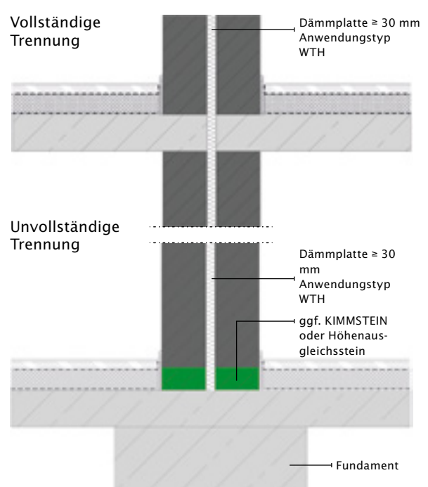
Schnitt
