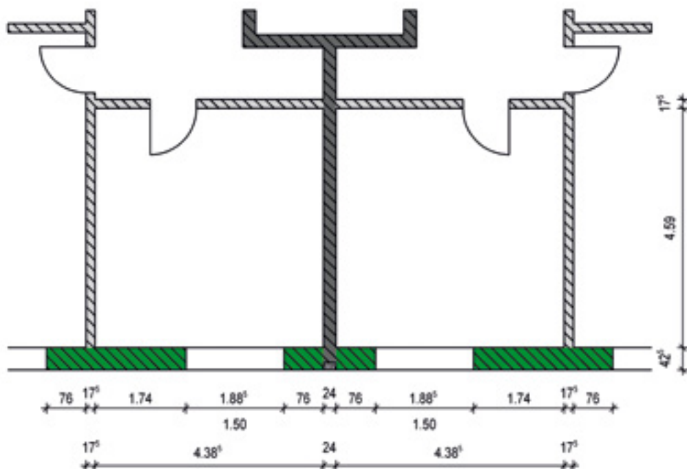
Bild 5.3: Grundriss zweier nebeneinander liegender Wohnräume.
