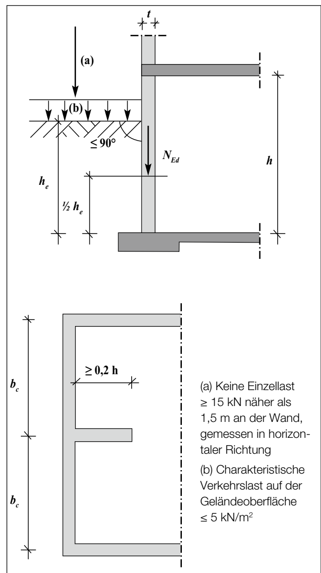
Bild 17: Variablen für Kellerwände in Schnitt und Grundriss.
