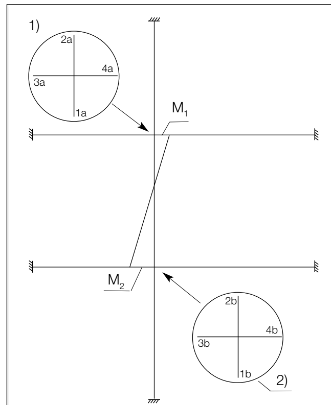
Bild 10: Vereinfachtes Rahmenmodell.
