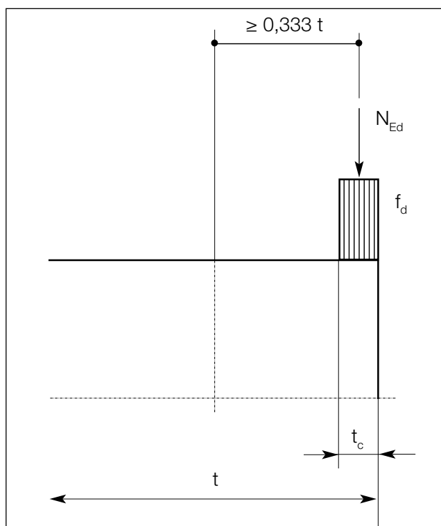
Bild 11: Ausmitte der Bemessungslast bei Aufnahme mit einem Spannungsblock.
