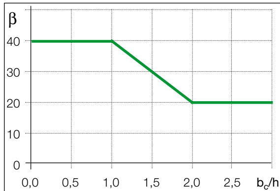
Bild 16: Faktor \beta in Abhängigkeit des Verhältnisses b_c/h
