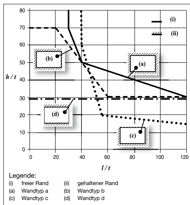
Bild 9: Minstdicke und Grenzabmessungen für nicht tragende innere Trennwände.
