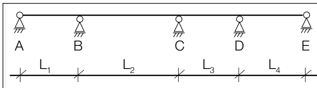
Bild 5: Berücksichtigung der Durchlaufwirkung bei der Ermittlung von Deckenauflagerkräften von einachsig gespannten Decken.
