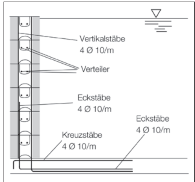
Bild 14: Bewehrungsanordnung
