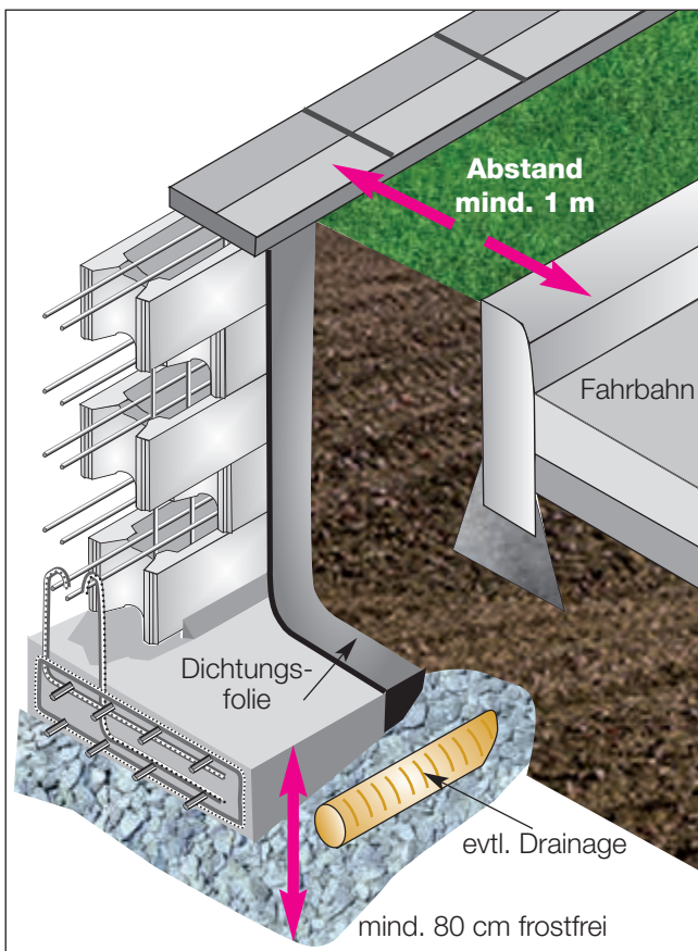
Bild 11: Winkelstützmauer (Schemaskizze)
