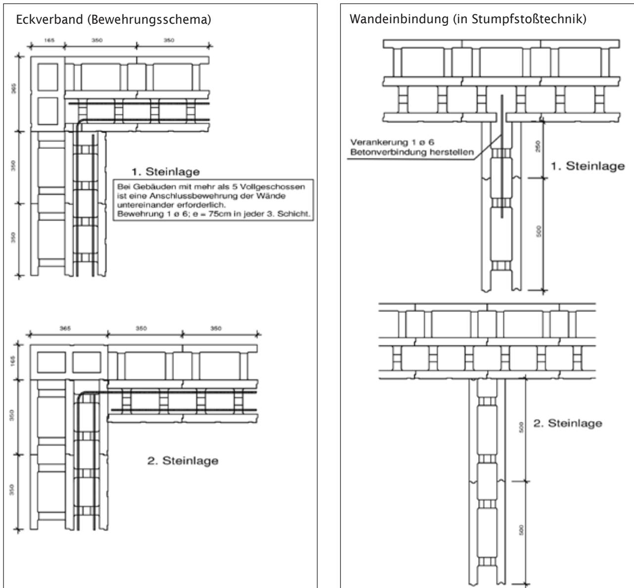
Bild 4: Bewehrungsschema Eck- und Wandeinbindung bei KLB Schalungssteinen mit Vorsatzschale
